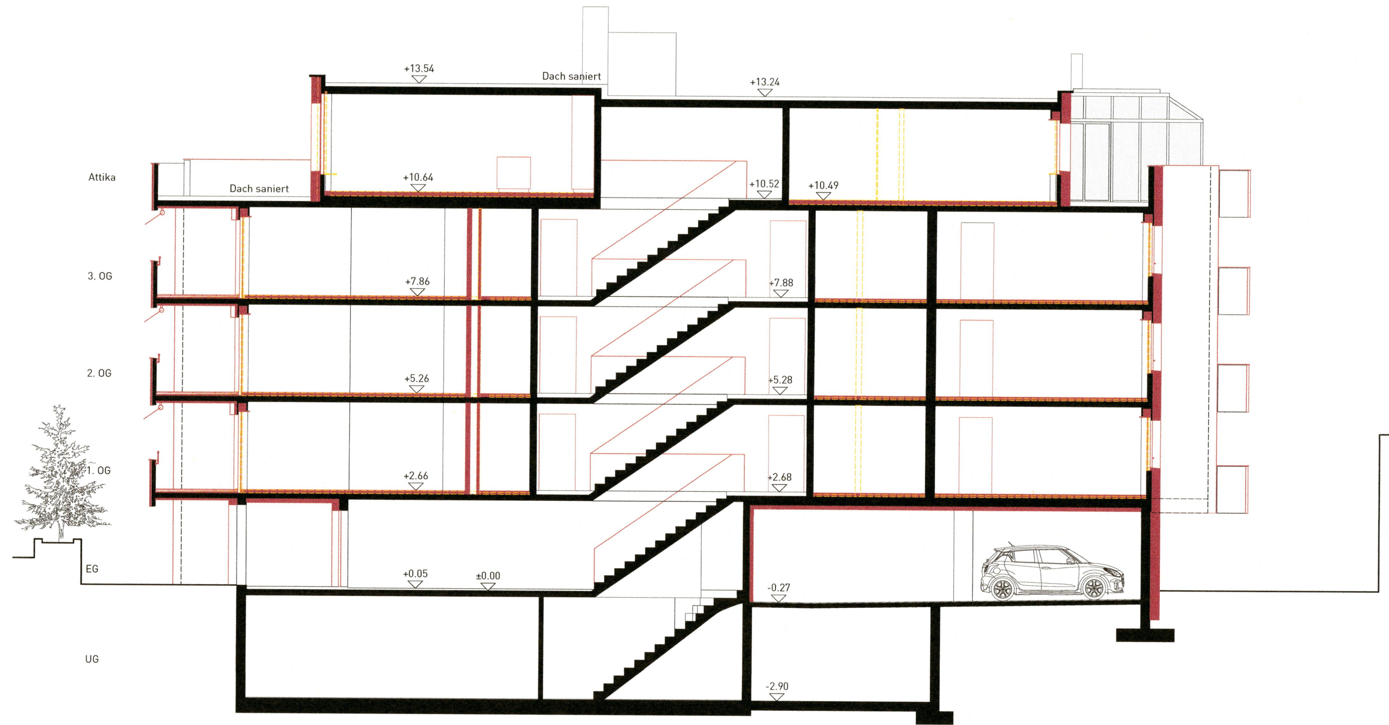
Gebäudeschnitt 1
