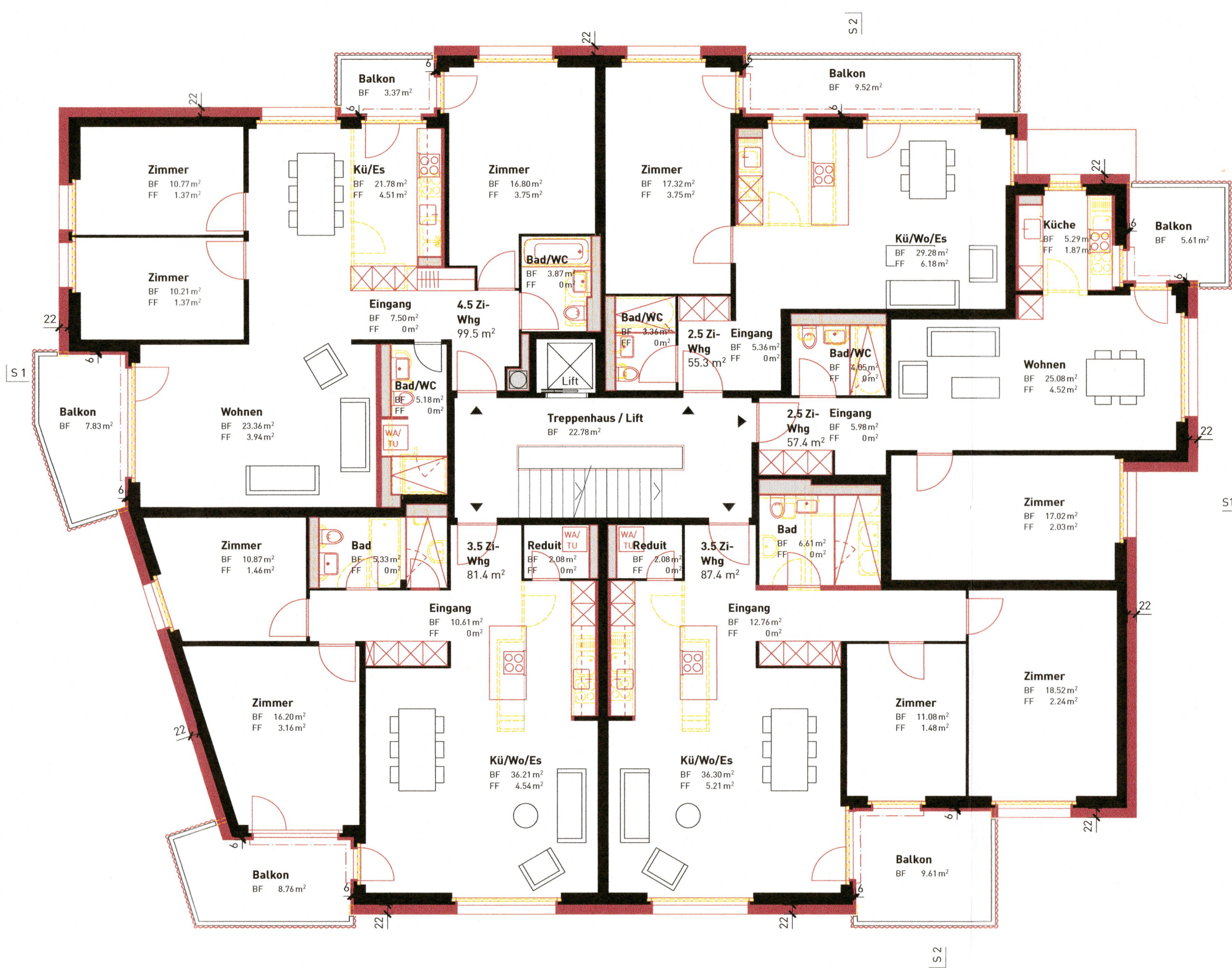
3. Obergeschoss
