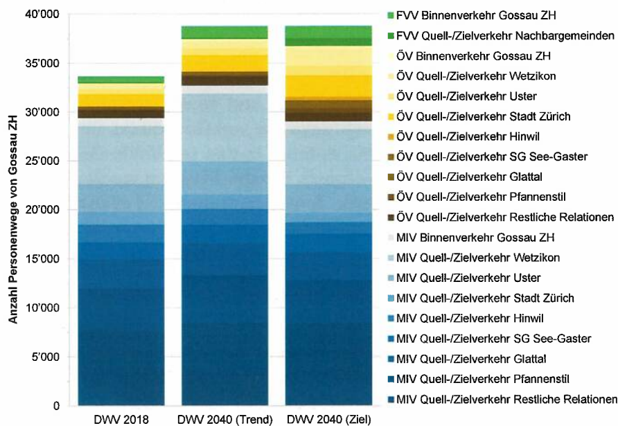
Abbildung 5 Verteilung der Personenwege des Quell-, Ziel- und Binnenverkehrs von Gossau auf die Verkehrsmittel und räumliche Relationen; Ist-Zustand, Prognose/Trend und Ziele (Basis: GVM-ZH, FVV ergänzt.)
