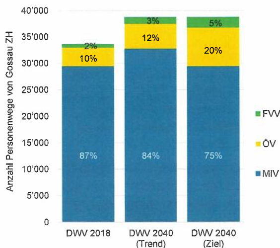
Abbildung 6 Modal Split des Quell-, Ziel- und Binnenverkehrs von Gossau (Personenwege nach Territorialprinzip); Ist-Zustand, Prognose/Trend und Ziele (Basis: GVM-ZH, FVV ergänzt).
