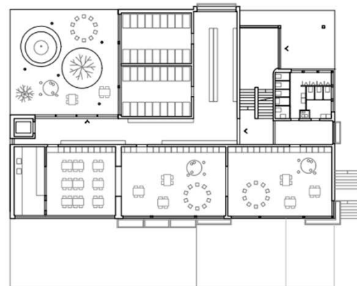
rez supérieur projet
