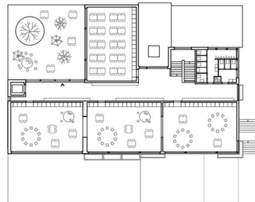
étage projet
