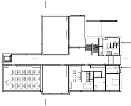
rez inférieur existant
