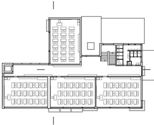
étage existant
