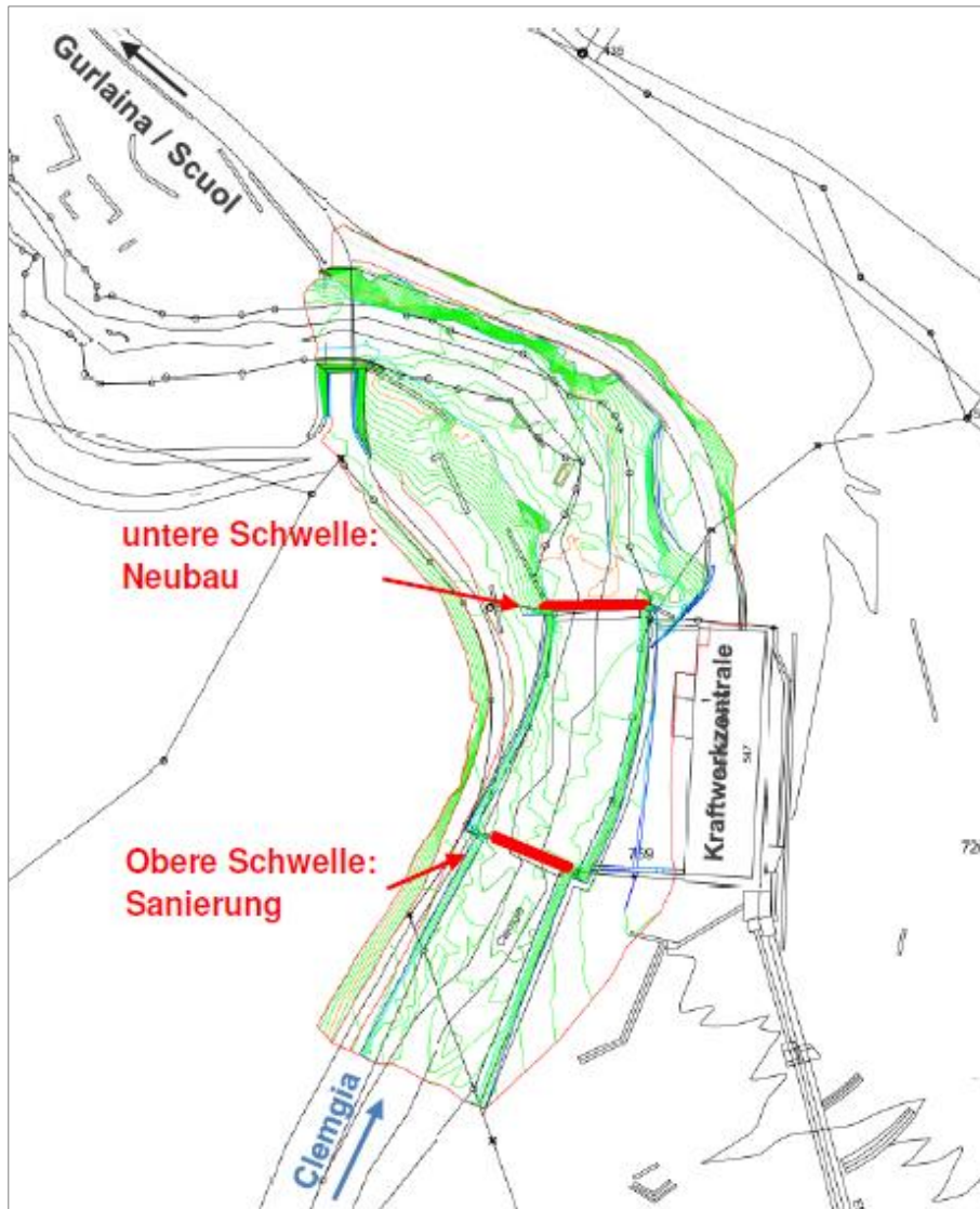
Verbauungen bei der Zentrale des Elektrizitätswerks Clemgia
