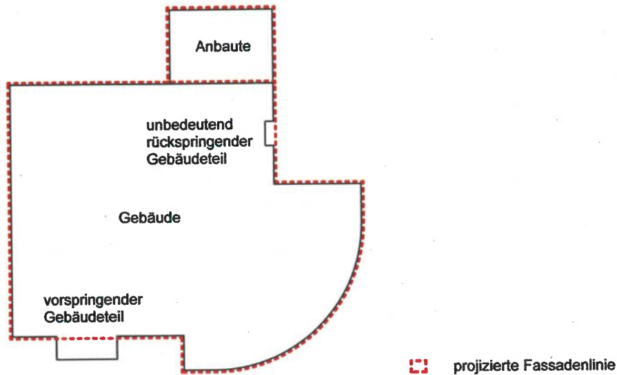
Figur 3.3 Projizierte Fassadenlinie
