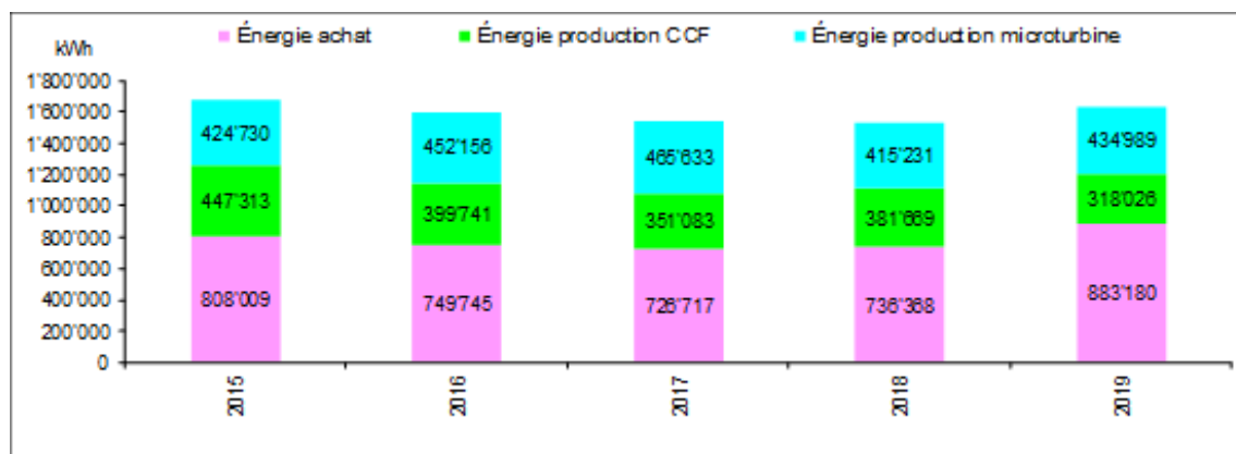
Figure 6 : Bilan électrique
