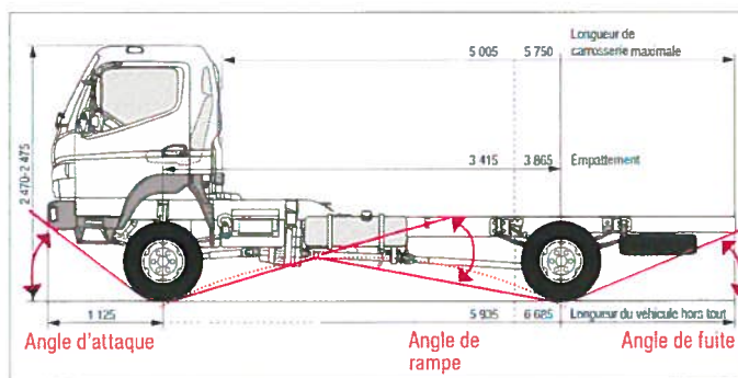
Mitsubishi Fuso Canter 4x4, modèle 6C18 équipé pour le service hivernal
