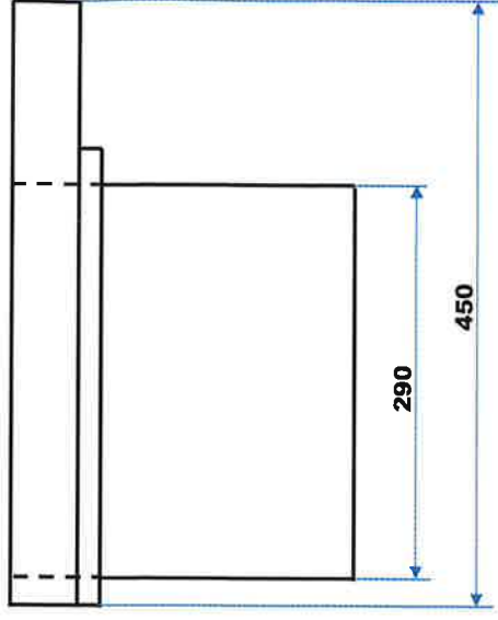
Vue Sud
