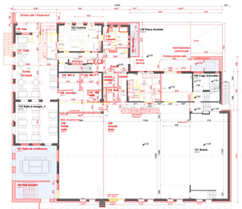
Etape 2 Plan du rez-de-chaussée
