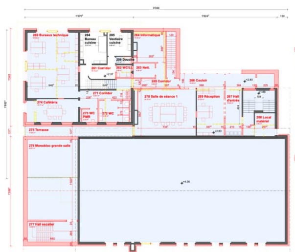
Etape 2 Plan du 1er étage
