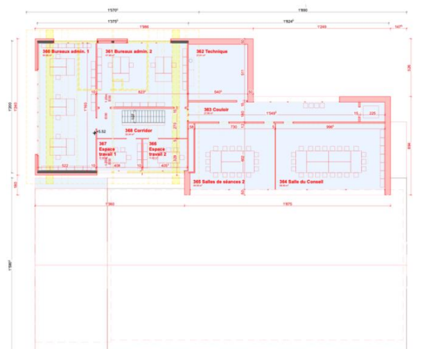
Etape 2 Plan du 2ème étage
