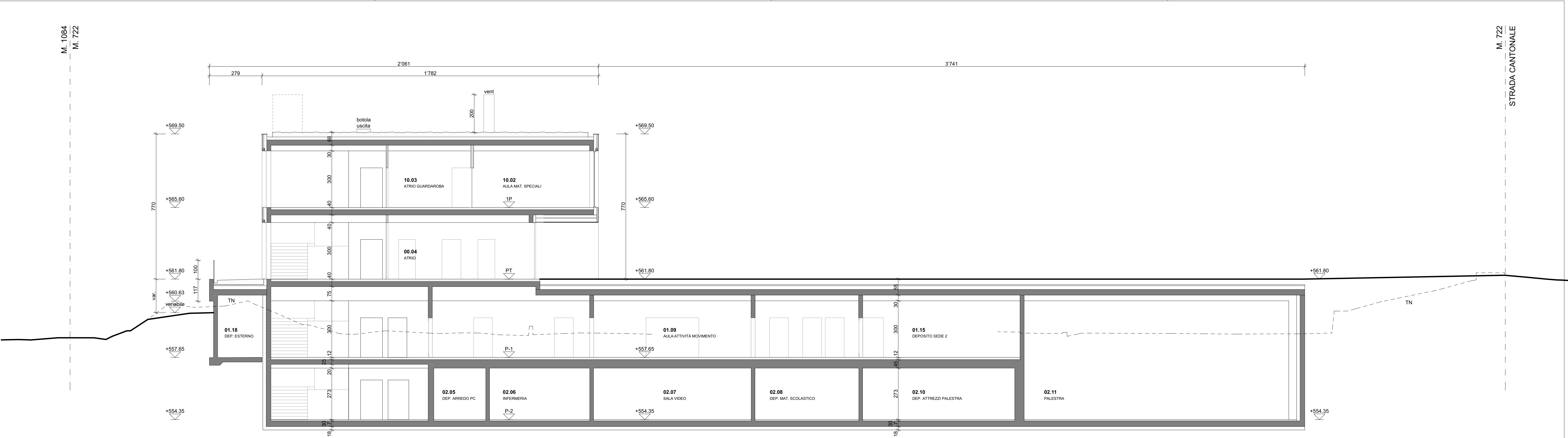
SEZIONE 6
