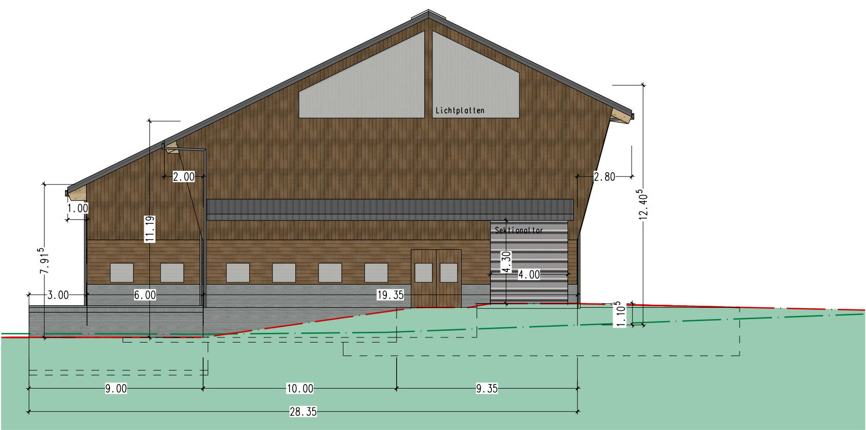
Fassade Ost
