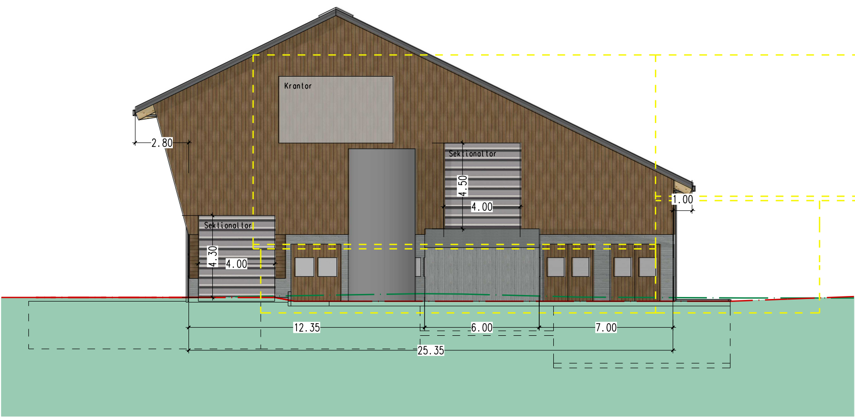
Fassade Ost
