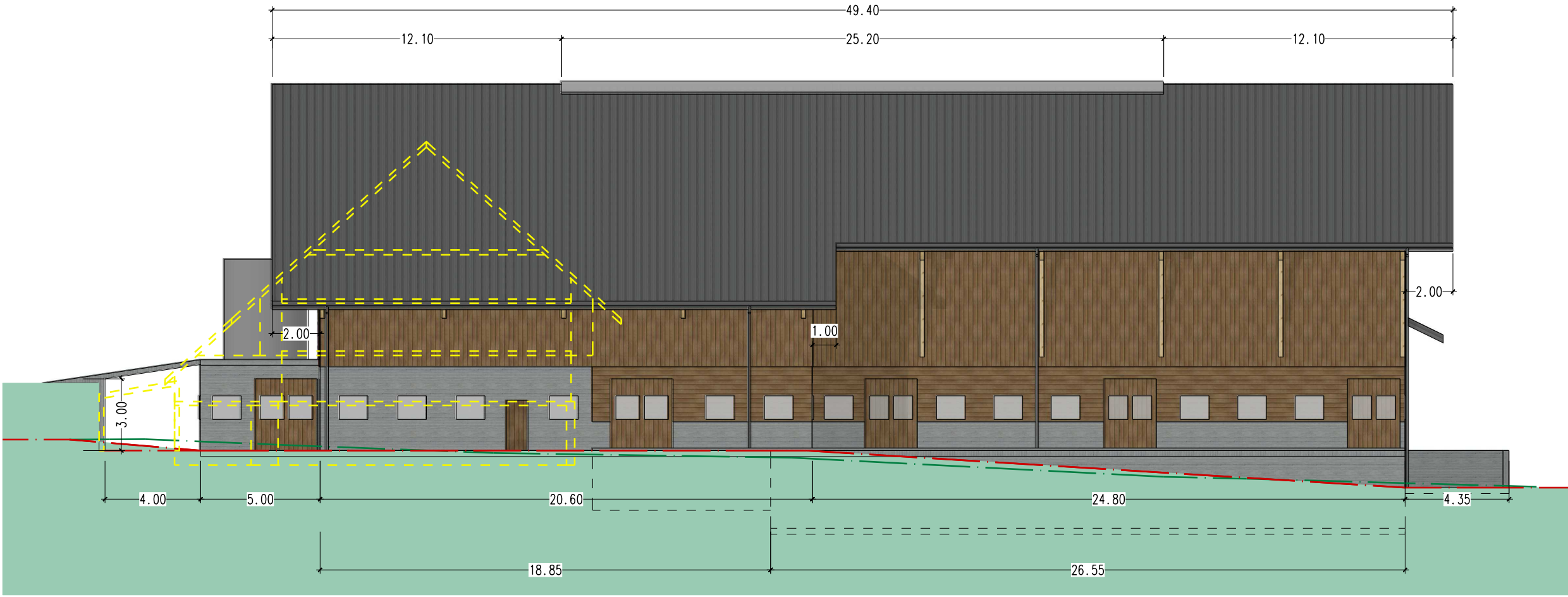
Fassade Süd
