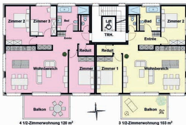
Überbauung Dorfmatte Marbach im Grundriss.
