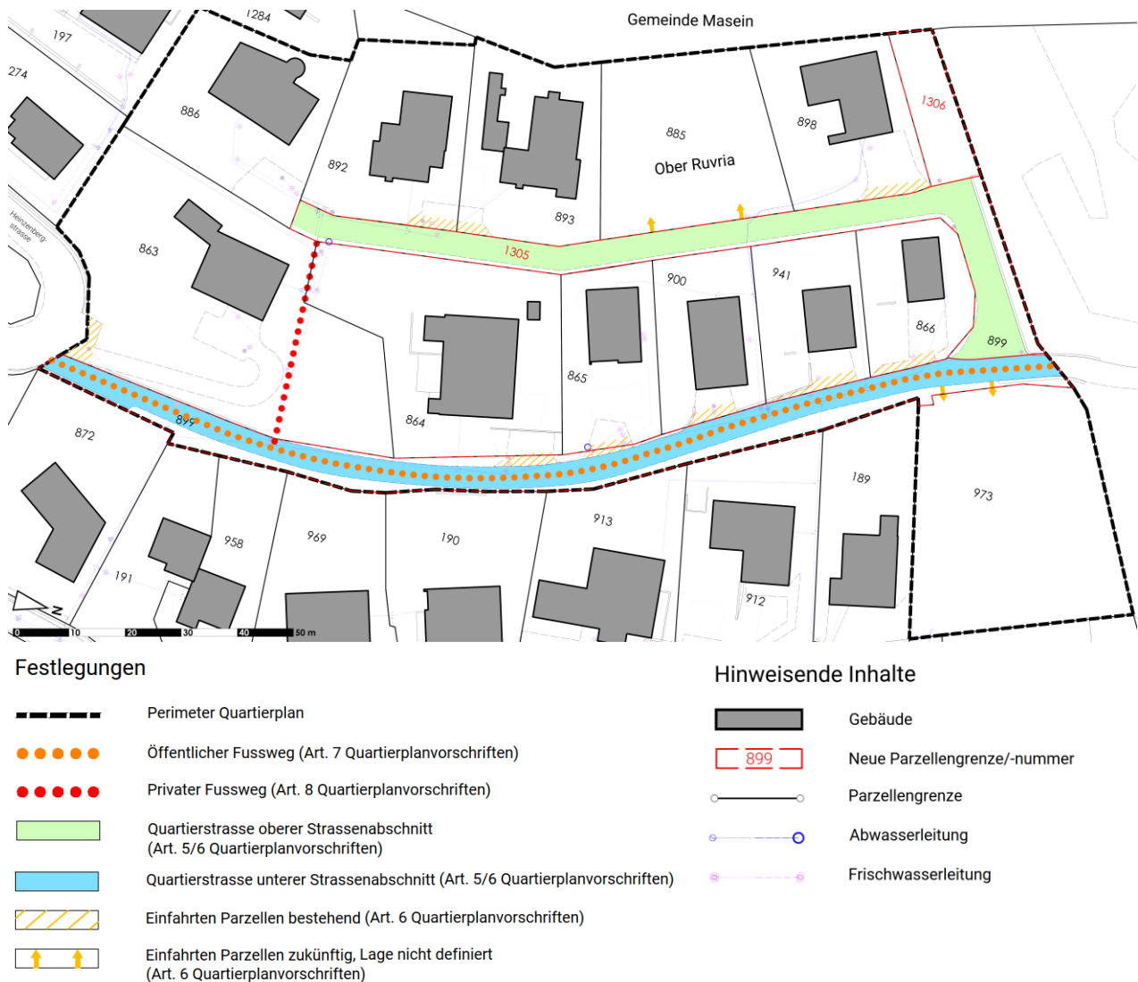
Abb. 6: Quartiererschliessungsplan Ober Ruvria mit Landumlegung (eigene Darstellung)
