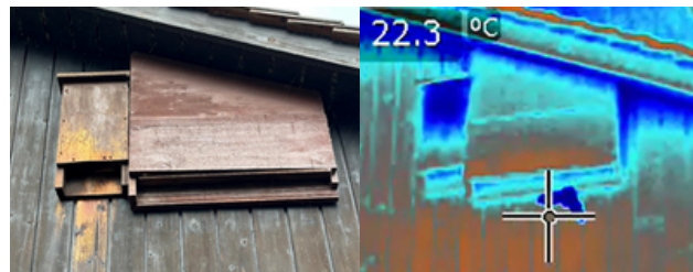
Fledermauskasten an der Ostfassade des Zieglerhauses bei Tageslicht (links) und Ausflug einer Fledermaus aus dem Kasten, aufgenommen mit einer Wärmebildkamera in der Nacht (rechts). Fotos: Sarah Wettstein (links) und Marc Van den Bergh (rechts)
