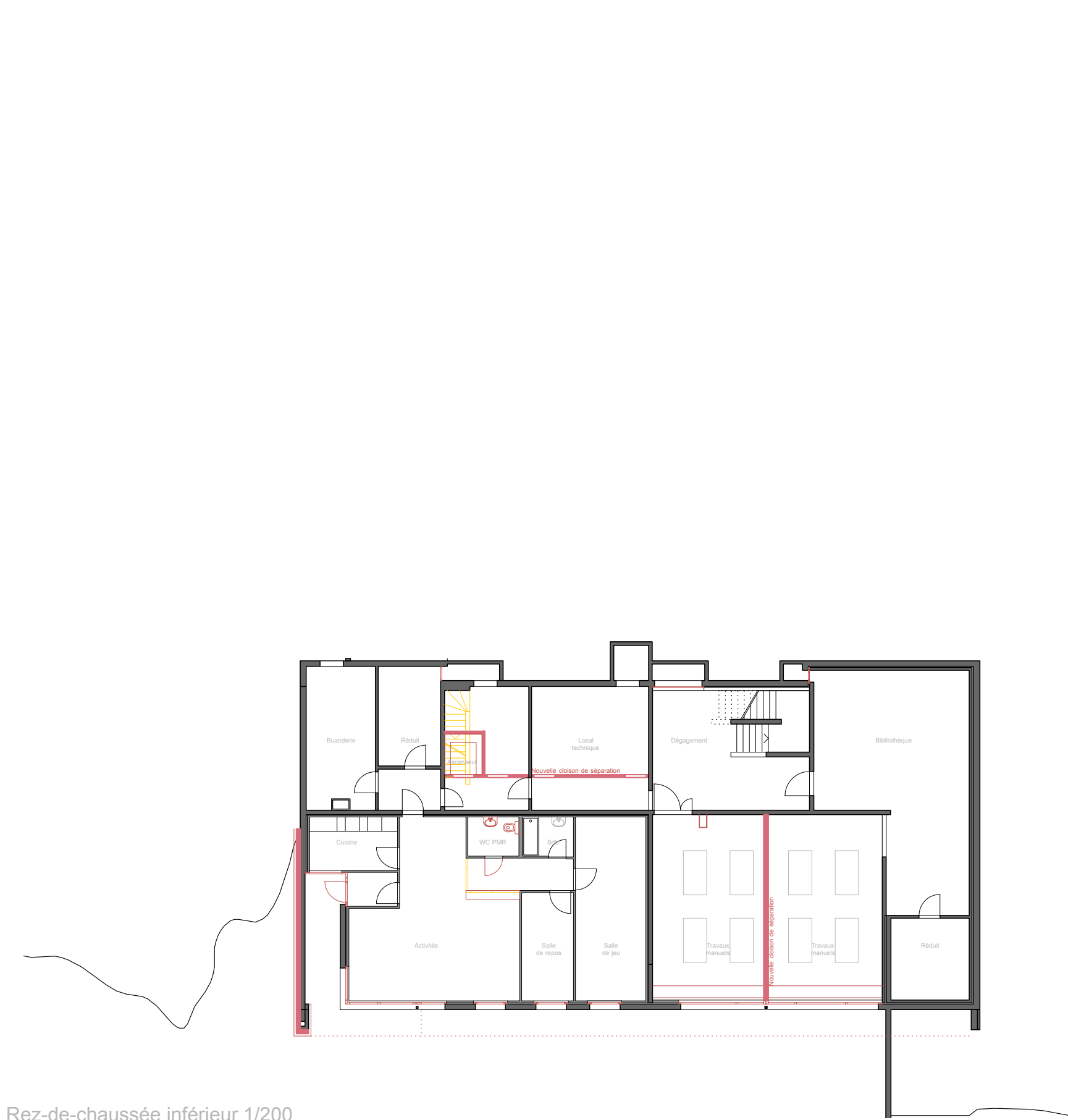
Rez-de-chaussée inférieur 1/200
