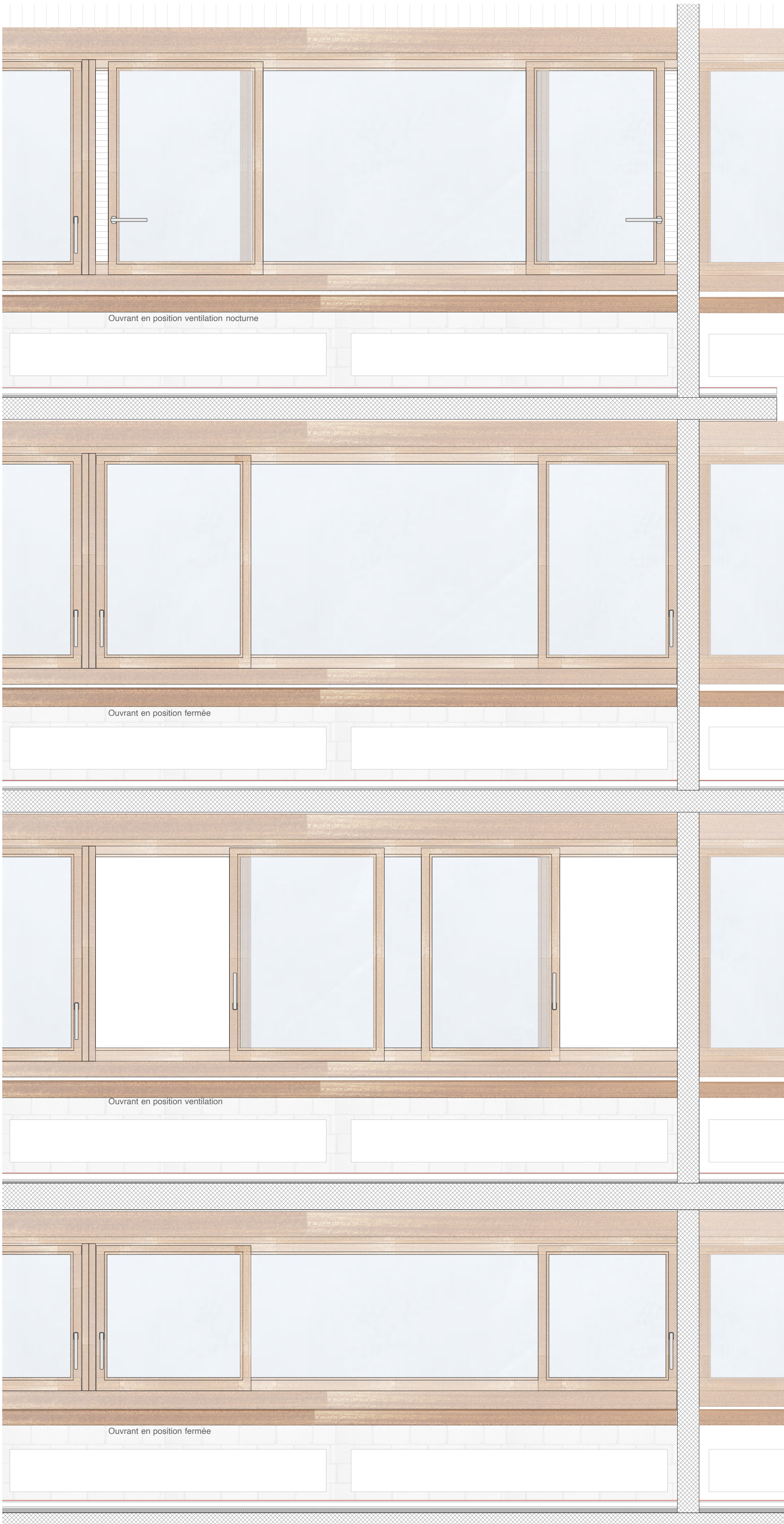
Élévation intérieure Salles de classe 1/20
