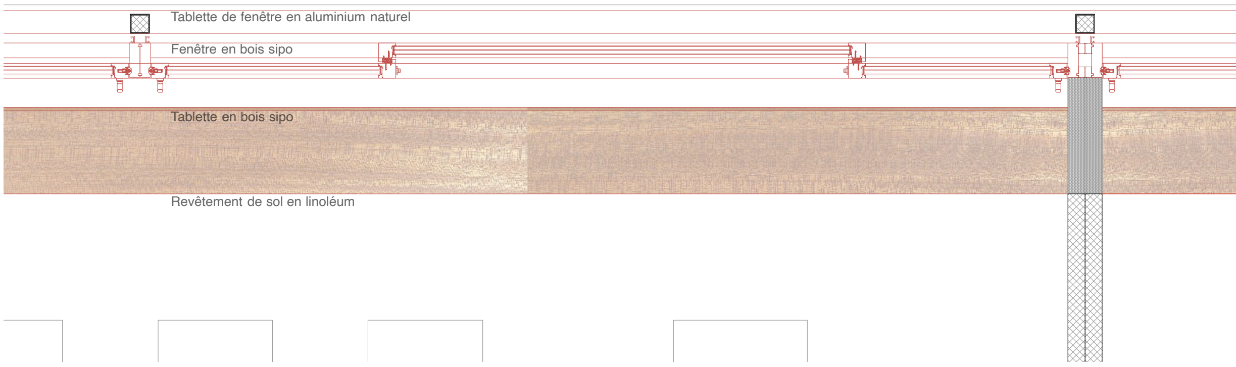
Plan façade Sud Salle de classe 1/20
