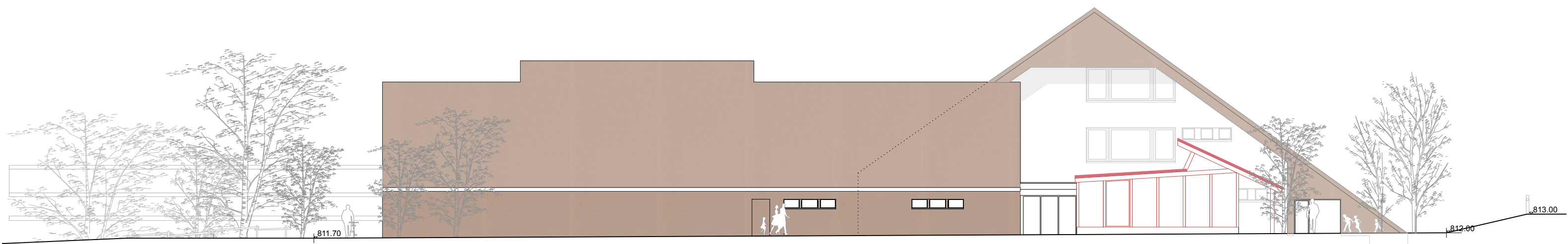
Élévation Nord 1/200
