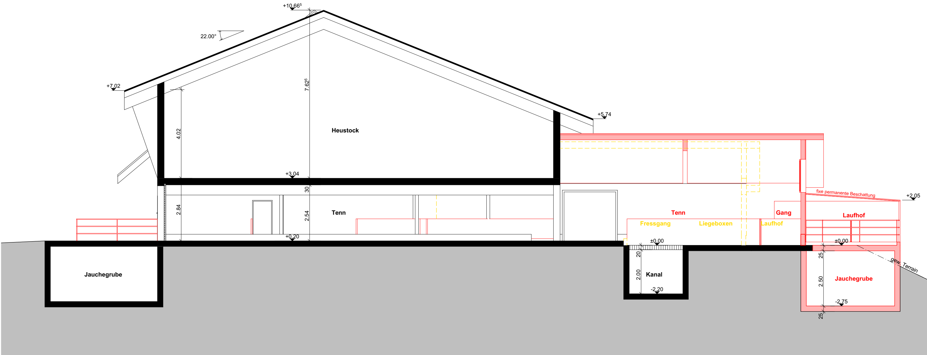
Schnitt B-B
