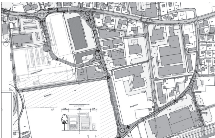
Ausschnitt aus Erschliessungskonzept Industriegebiet Usserhirschland
