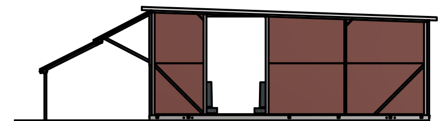
Ostfassade 1:75
