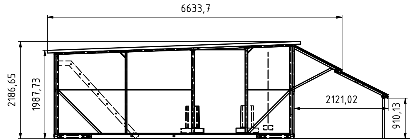
Querschnitt 1:50
