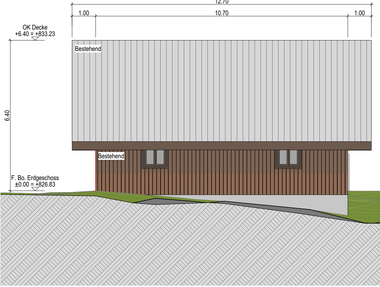
Ostfassade
