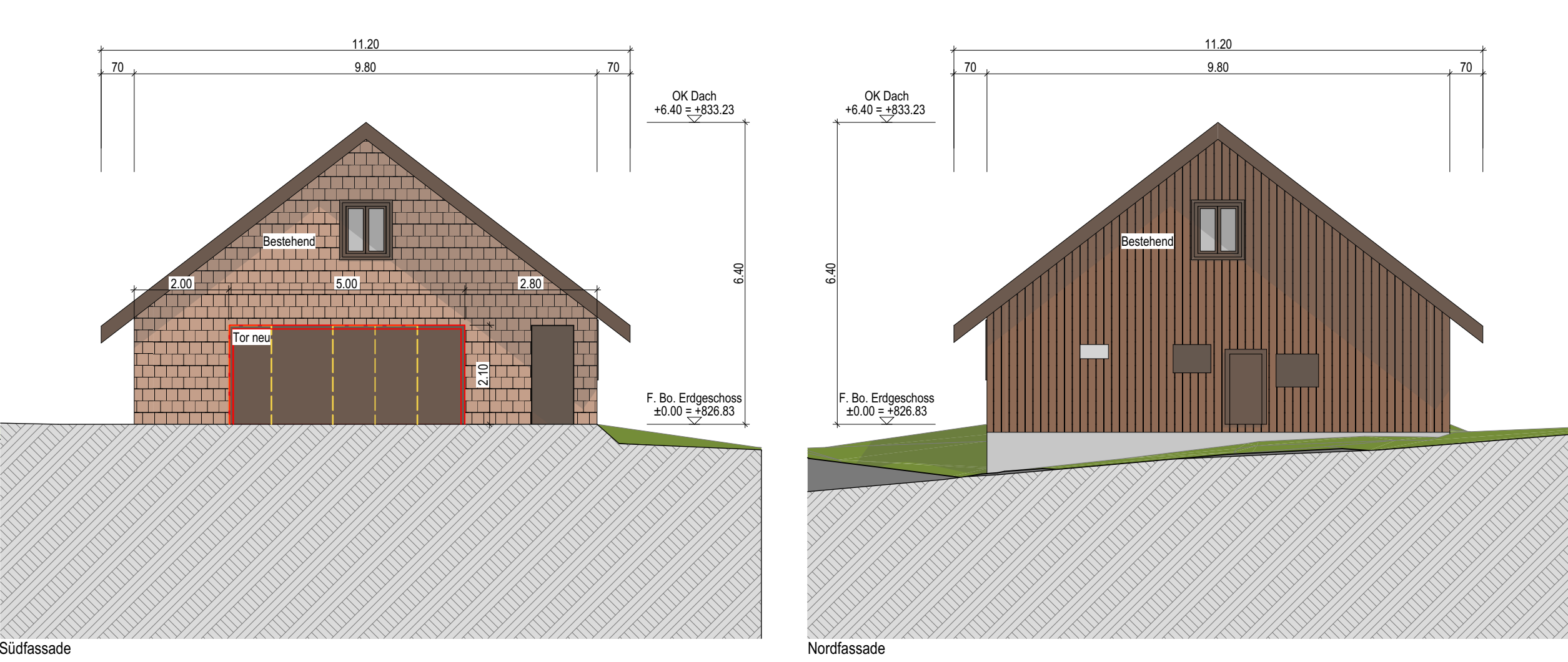
Südfassade
