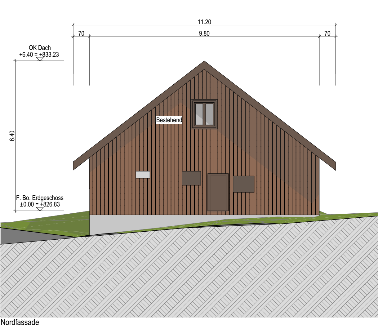
Nordfassade
