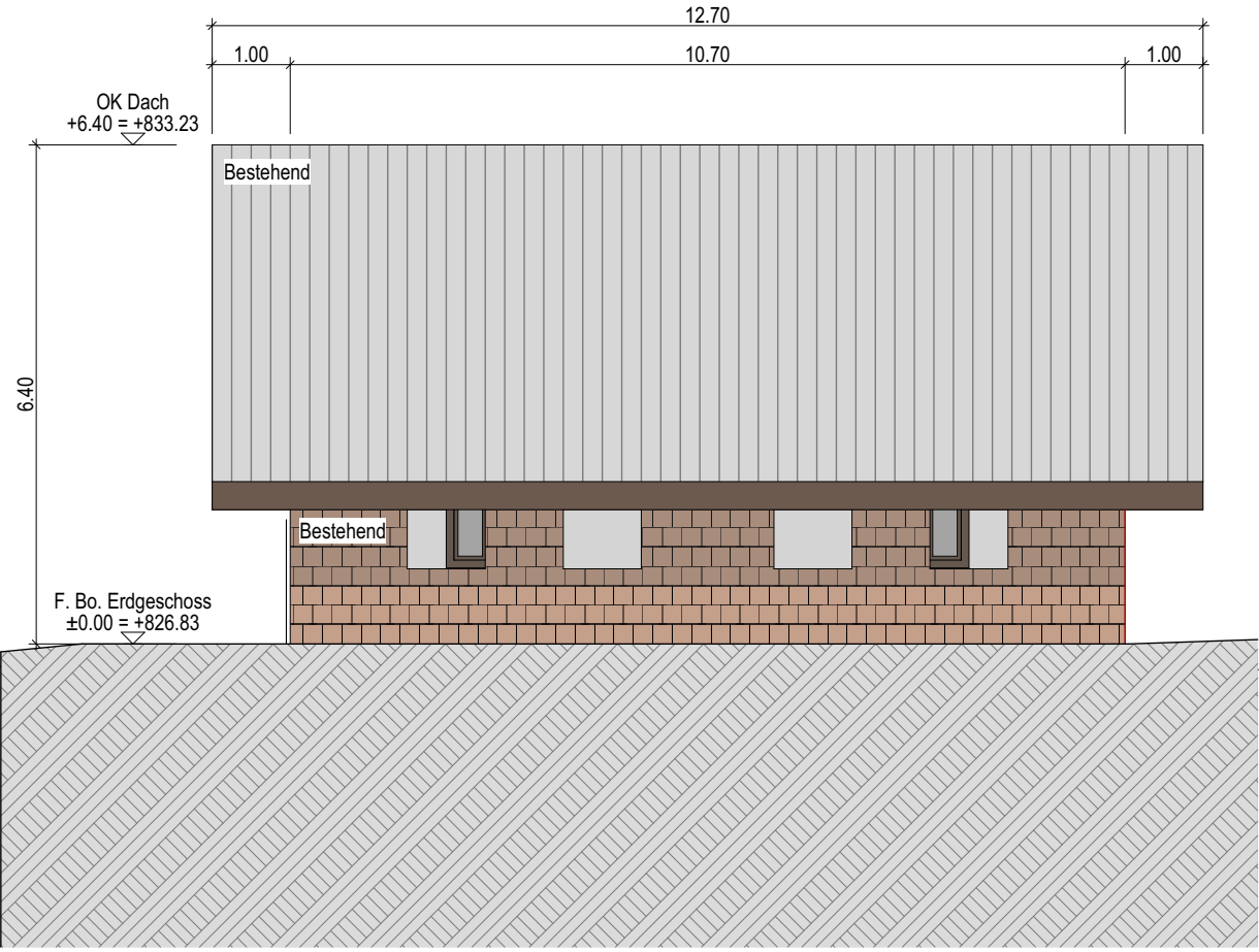
Westfassade
