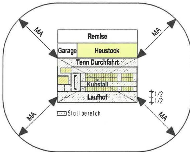
Abb. 3: Mindestabstand (=Hüllkurve) um ein Stallgebäude für Rindvieh mit nicht emittierenden Gebäudeteilen.
