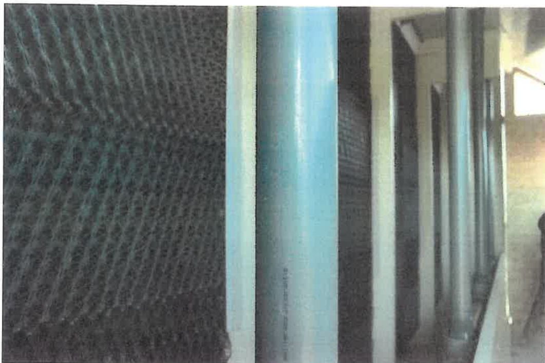
Abbildung 1: Kunststoffwaben einer Abluftreinigungsanlage. Ansicht in der Druckkammer (Bild uwe).
