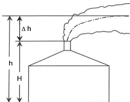
Abb. 12: Schema effektive Quellhöhe h , Höhe Abluftaustritt über Erdboden H , Abluftfahnenüberhöhung \Delta h
