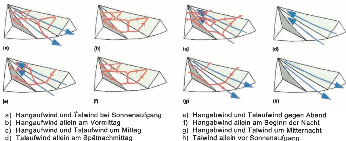
Abb. 7: Entwicklung der Hang- und Talwinde im Laufe eines Tages (Liljequist u. Cihak, 1979).
