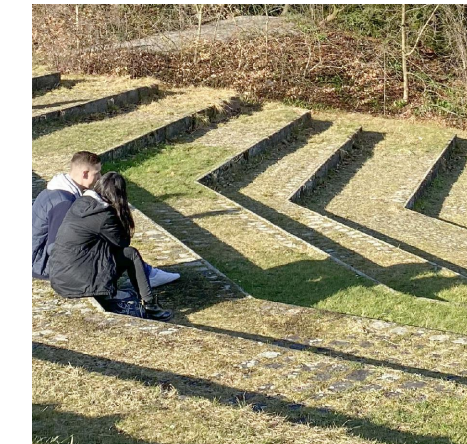
Sitzstufen entlang Böschung Granitstellplatten / Guber Bindersteine
