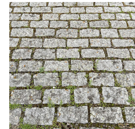
Parkfelder mit sickerfähigem Belag Granit Bindersteine 12, offene Fugen
