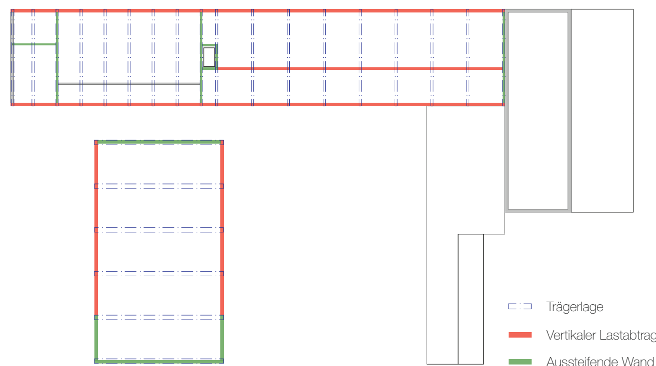
SCHEMA STATIK 1-500
