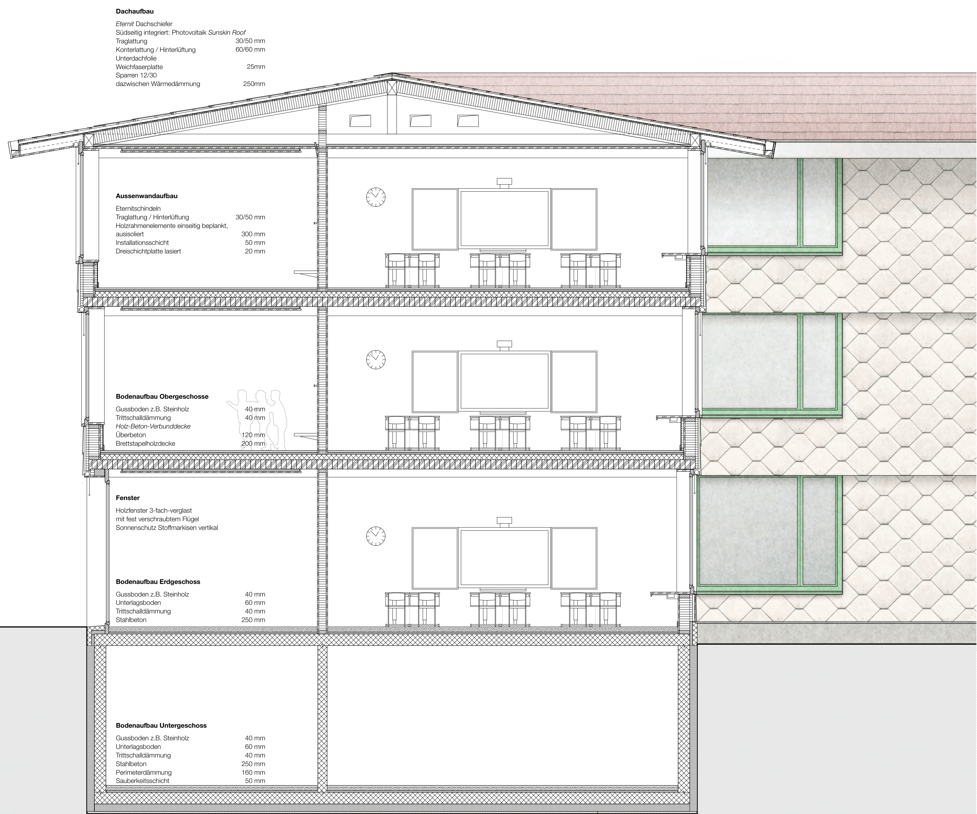
KONSTRUKTIONSSCHNITT 1-50
