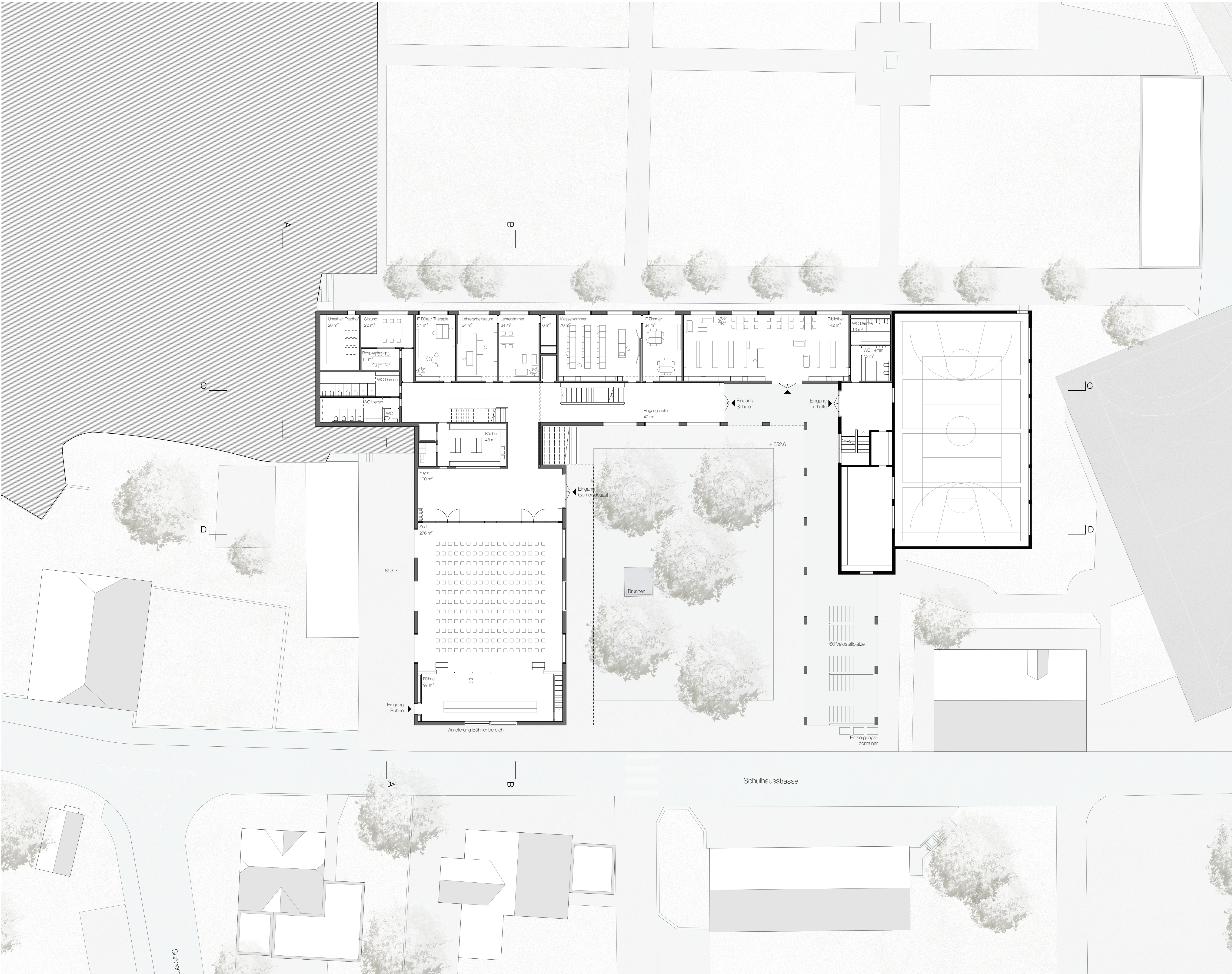
GRUNDRISS EG 1-200
