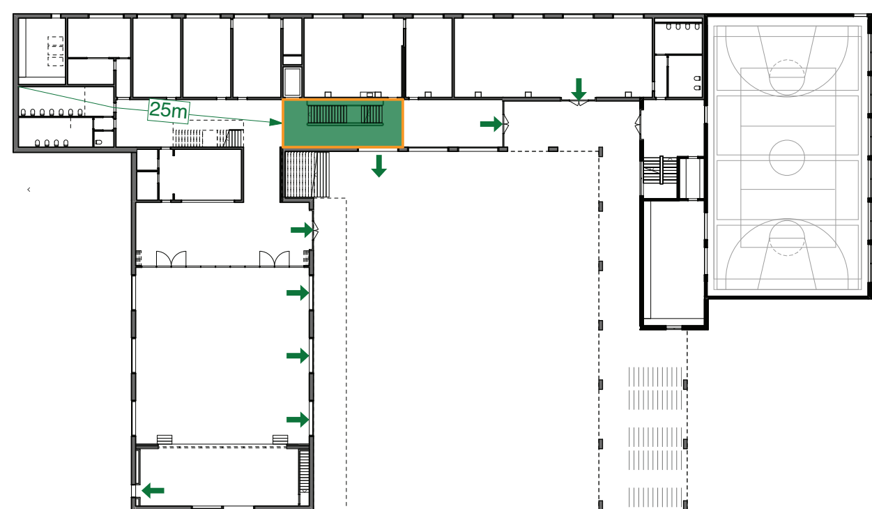
SCHEMA BRANDSCHUTZ EG 1-500
