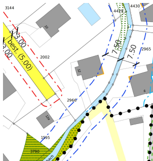
Auszug Strassen- und Baulinienplan nach OPR
