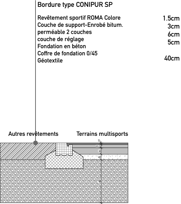
Coupe type bordure
